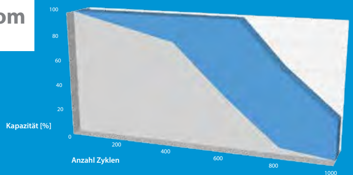
Kapazität des SP8000-12 im Vergleich zum Original
